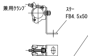
④ 側固定用クランプ
