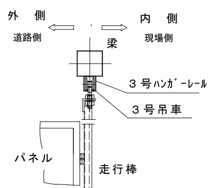
梁、走行棒、吊車 関連図
