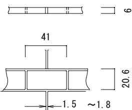
③ M4クランプ
