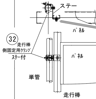
② 走行棒端部 取り付け要領図
